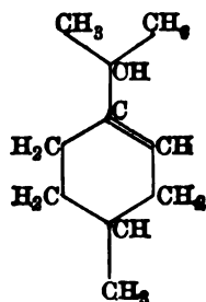
Menthene.
